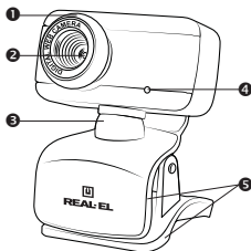
Joon. 1. Veebikaamera ehitus
